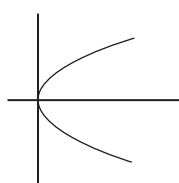
(b) Parabola
